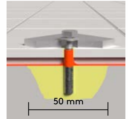
FIGUR 5. Kappilärbrytare
