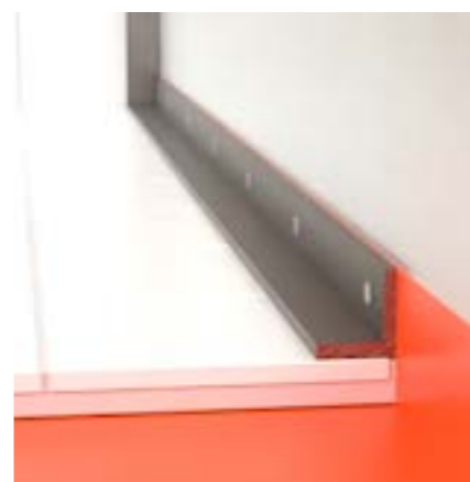
FIGUR 10. Mekanisk förankring av tätskikt.
