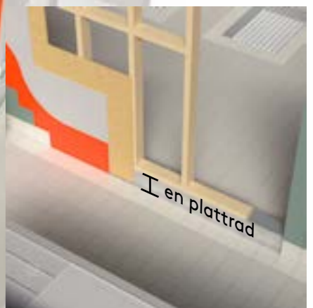
FIGUR 6. Kombinationsvägg
